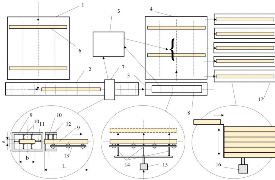
Рисунок 1. Схема линии сортировки пиломатериалов по плотности
