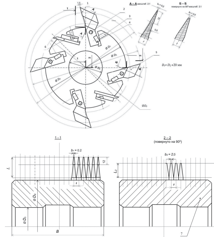
Рисунок 2. Конструкция полезной модели сборной фрезы по патенту № 229258
