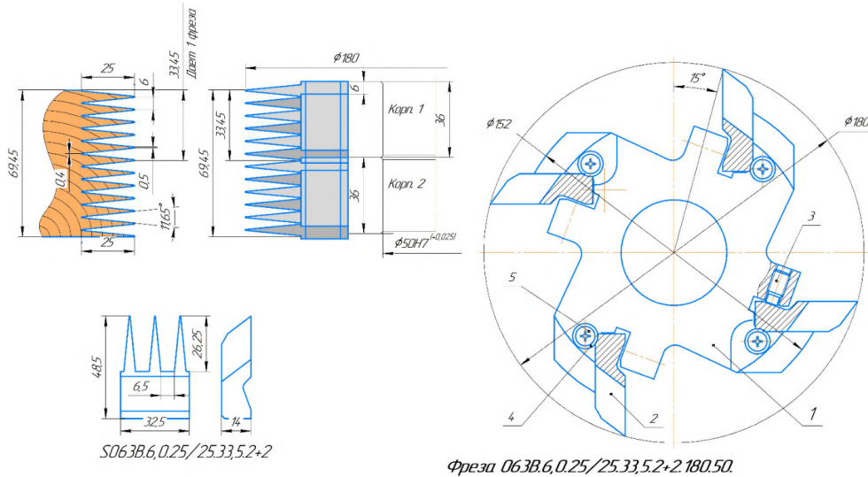
Рисунок 3. Конструкция фрезы с параметрами шипов по ГОСТ 19414–2023
