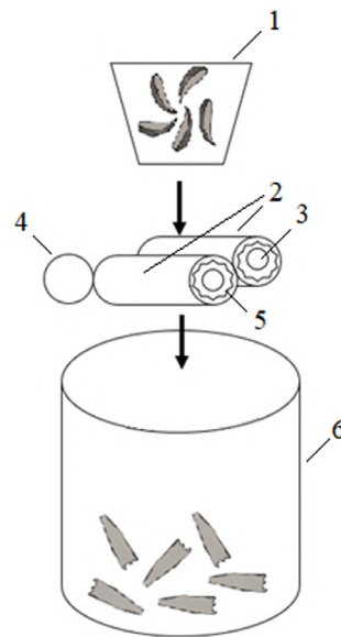
1 – емкость для предварительной подготовки лузги; 2 – валки; 3 – механизм регулировки просвета между валками; 4 – электродвигатель; 5 – ведущая и ведомая шестерни; 6 – бункер для приема уплощенной лузги
