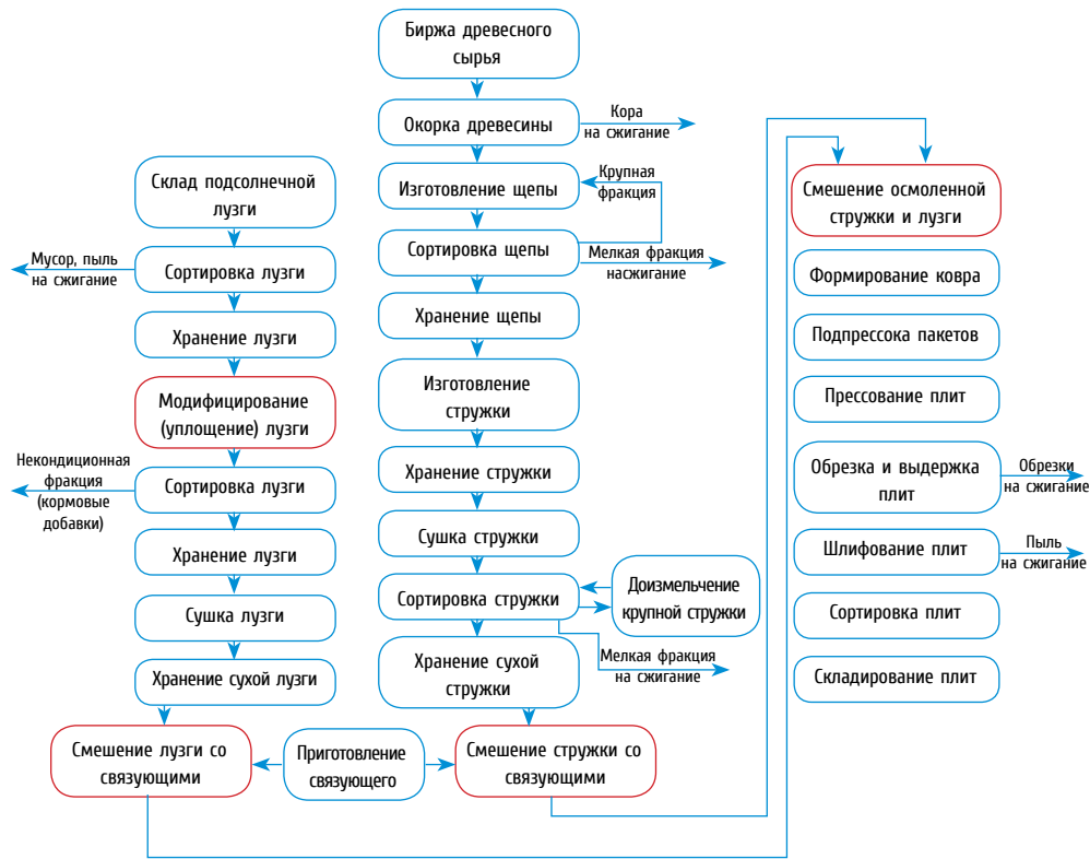
Рисунок 4. Технологическая схема производства древесно-лузговых плит
