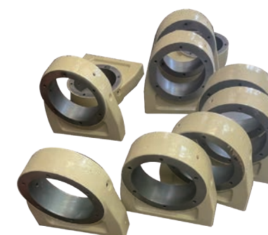
Подшипниковый
