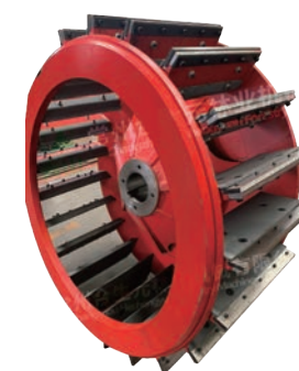
Импеллер
