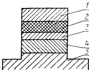
1 — медный стержень; 2 — образец испытуемый; 3 — пластина ков-тактная; 4 — пластина; 5 — основание
