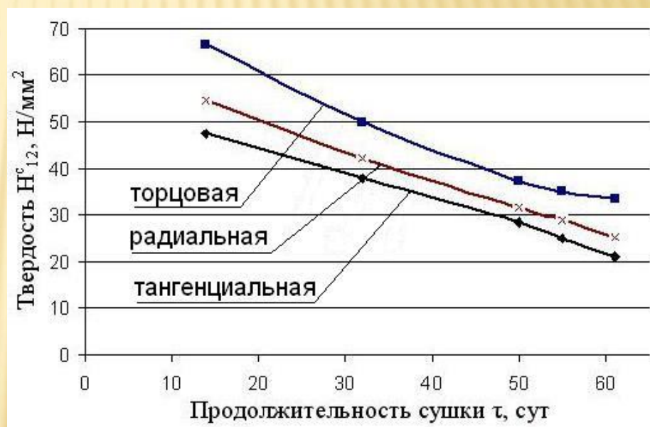
Статическая твердость
